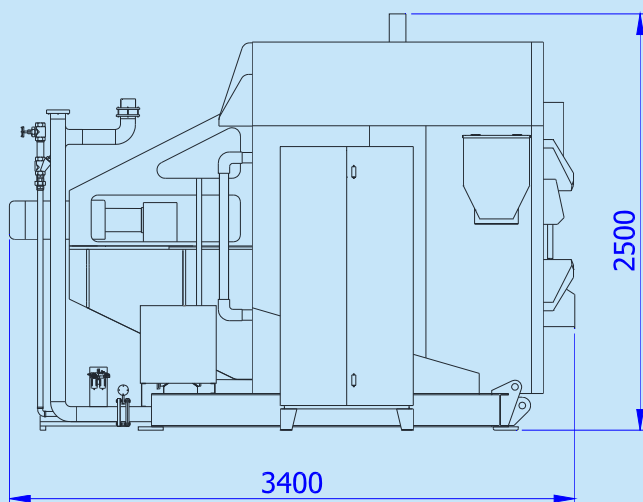
Wassar 360 機身尺寸圖 Machine Size(mm)
