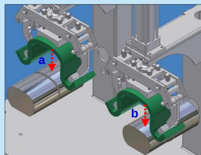
a. 熱壓狀態 Hot creasing status b. 冷壓狀態 Cold creasing status
